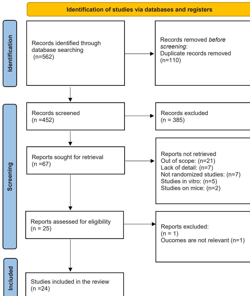
Fig. 1. Prisma Diagram.
